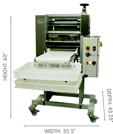
ADC250
